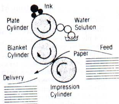
Offset Press
